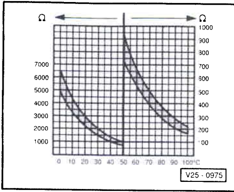
◀ Fig. 1 Valeurs de la résistance pour ♦ Transmetteur de température de liquide de refroidissement (G62) ♦ Transmetteur de température de l'air d'admission (G42)
