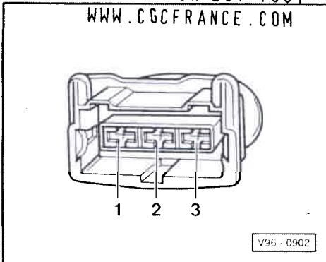
◀ Fig. 3 Bornage de la fiche à 3 pôles ♦ Fiche de détecteur de cliquetis 1 (G61)
